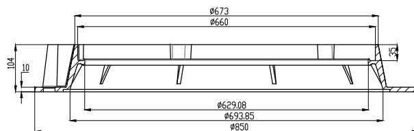
SEÇÃO C-C ESCALA 1 : 4
